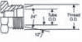
Male 24° Cone
